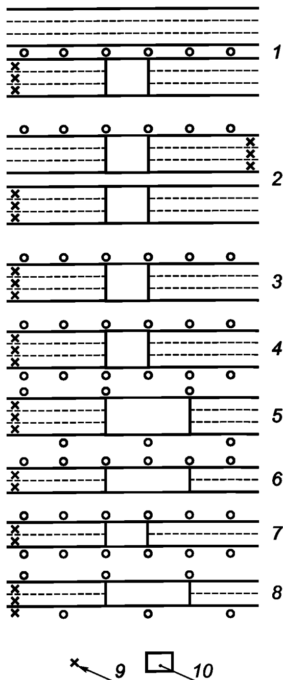
Рисунок Б.4 — Расположение контрольного участка при измерении средней освещенности улиц
