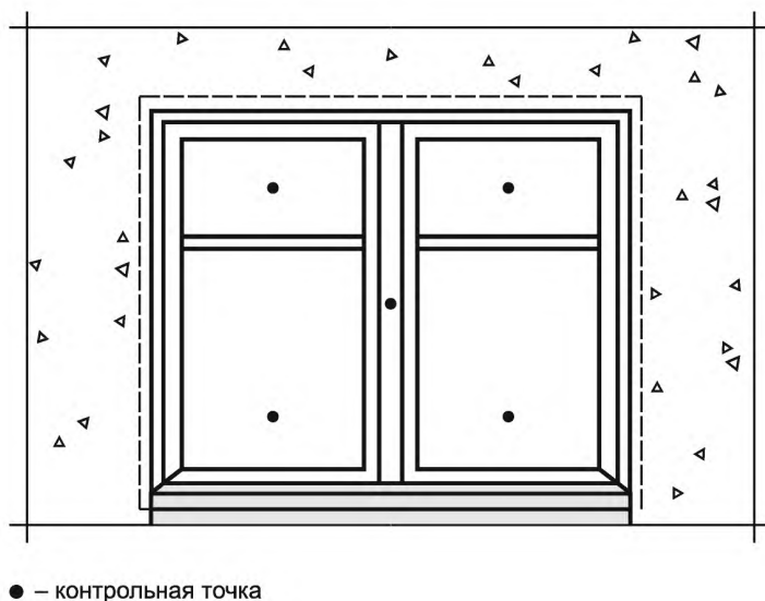
Рисунок Б.7 — Расположение контрольных точек на внешней поверхности окна при измерении вертикальной освещенности (засветки окон)
